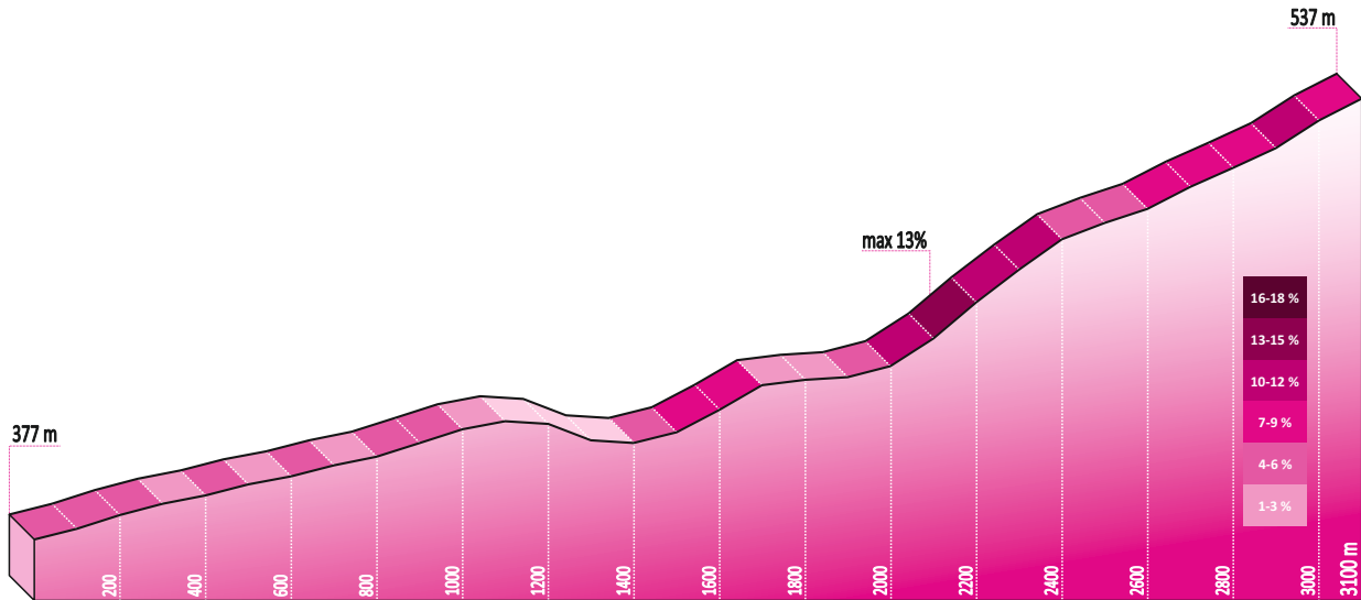
GPM Krásné Pole ↔3100 m ↗160m Ø5,2% max 13%
